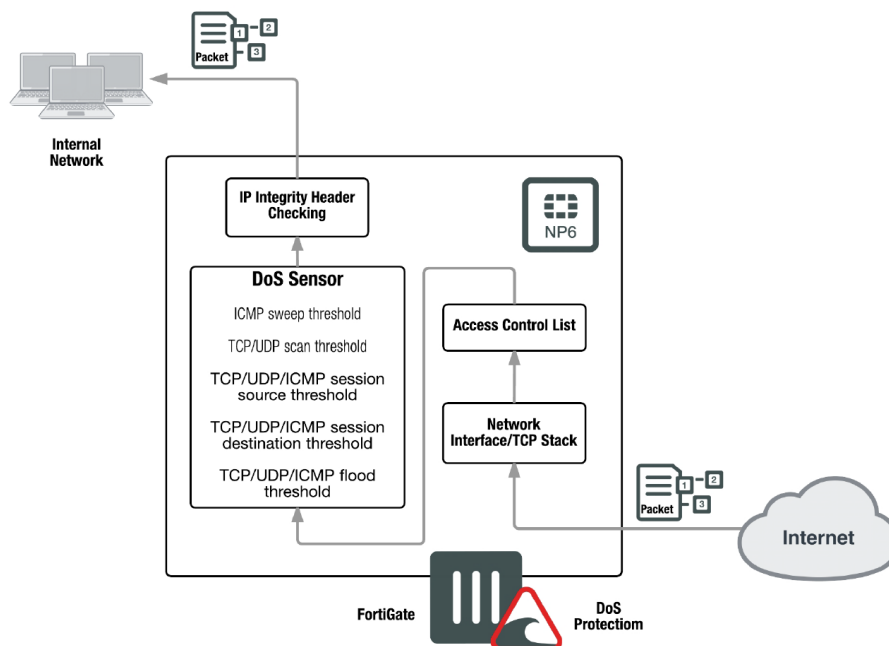
Figura 13.- Arquitectura NP6 en ataques DoS
